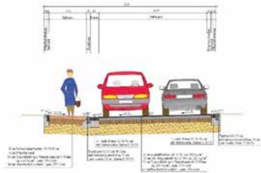
Regelquerschnitt innere Erschließungsstraße
