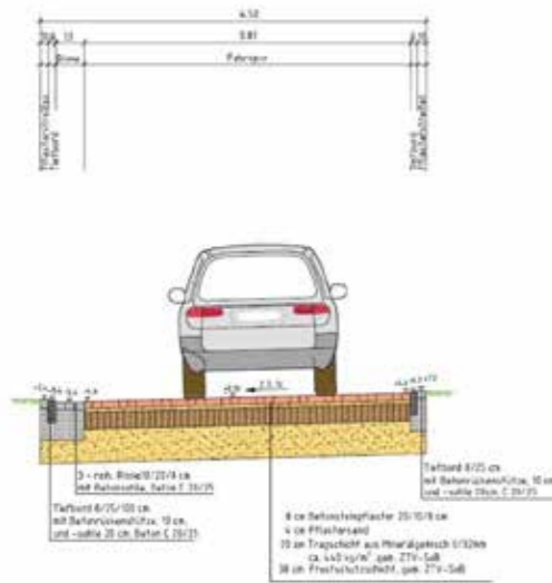
Regelquerschnitt Stichstraße
