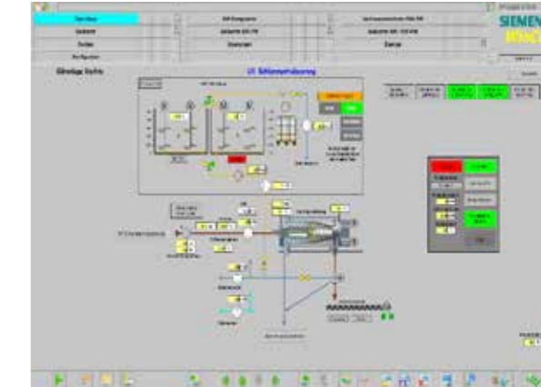
Bild: Prozessbild zu den Entwässerungsvorgängen
